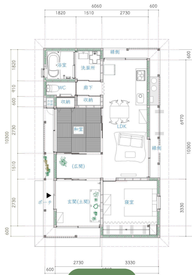
平面図 A
