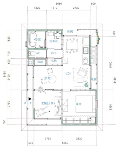
平面図 B
