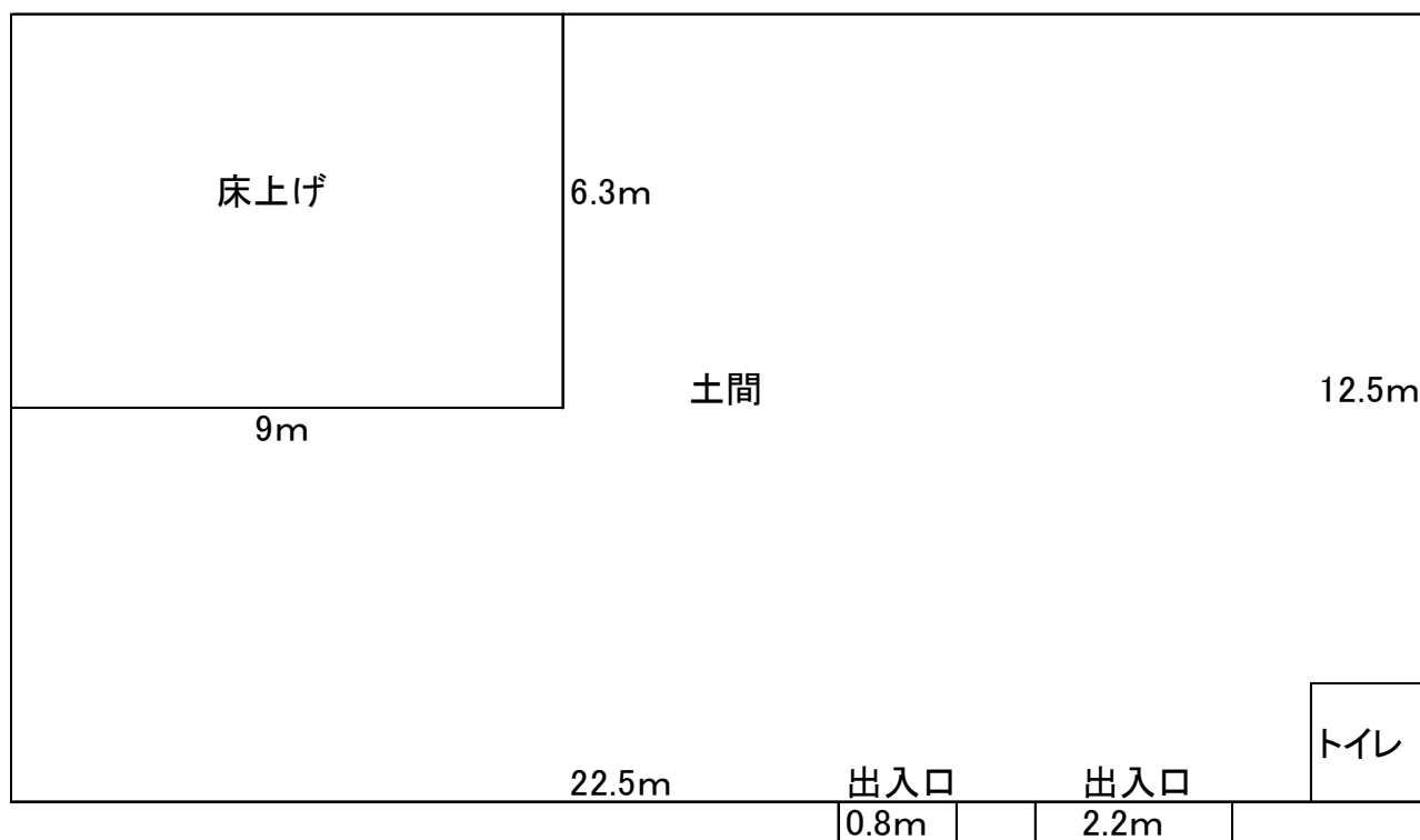
間取り図
