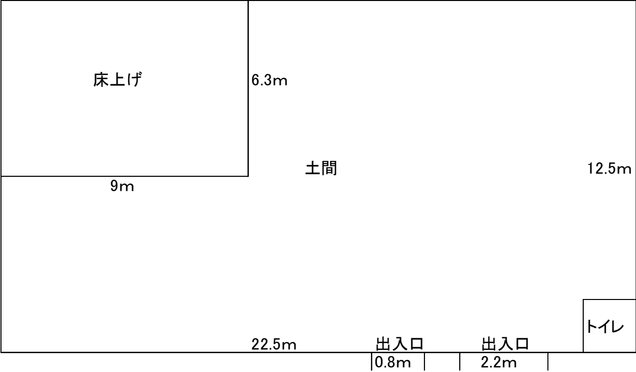
間取り図
