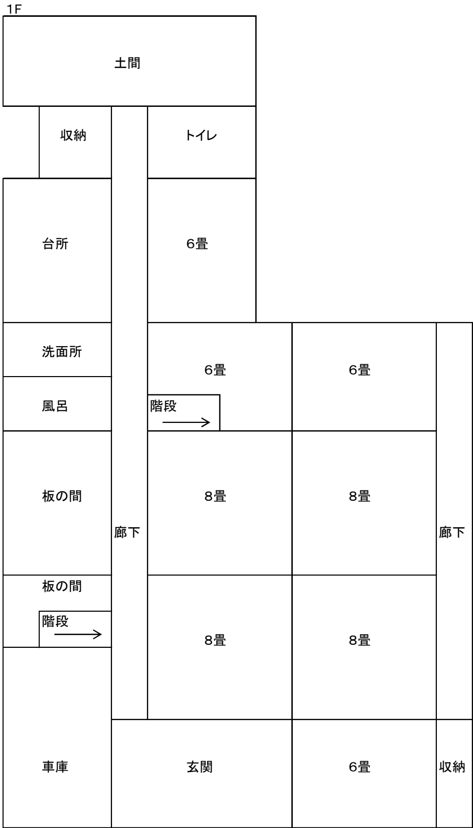
間取り図
