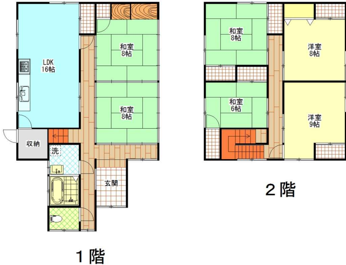
間取り図
