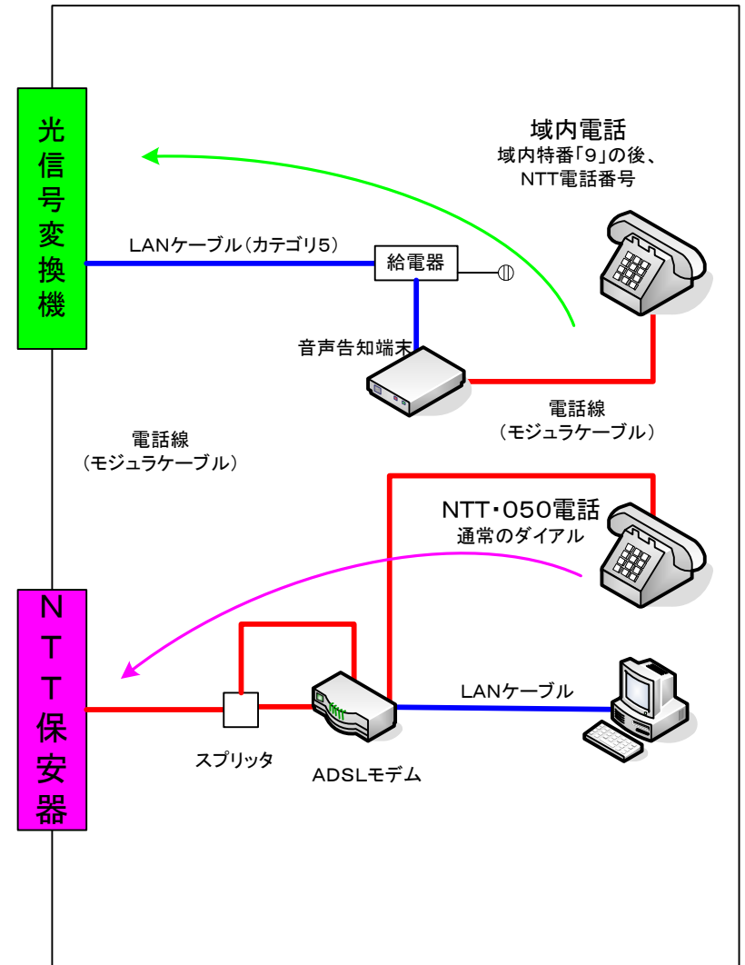
ADSL<050電話利用> (NTT・域内各専用電話の場合)
