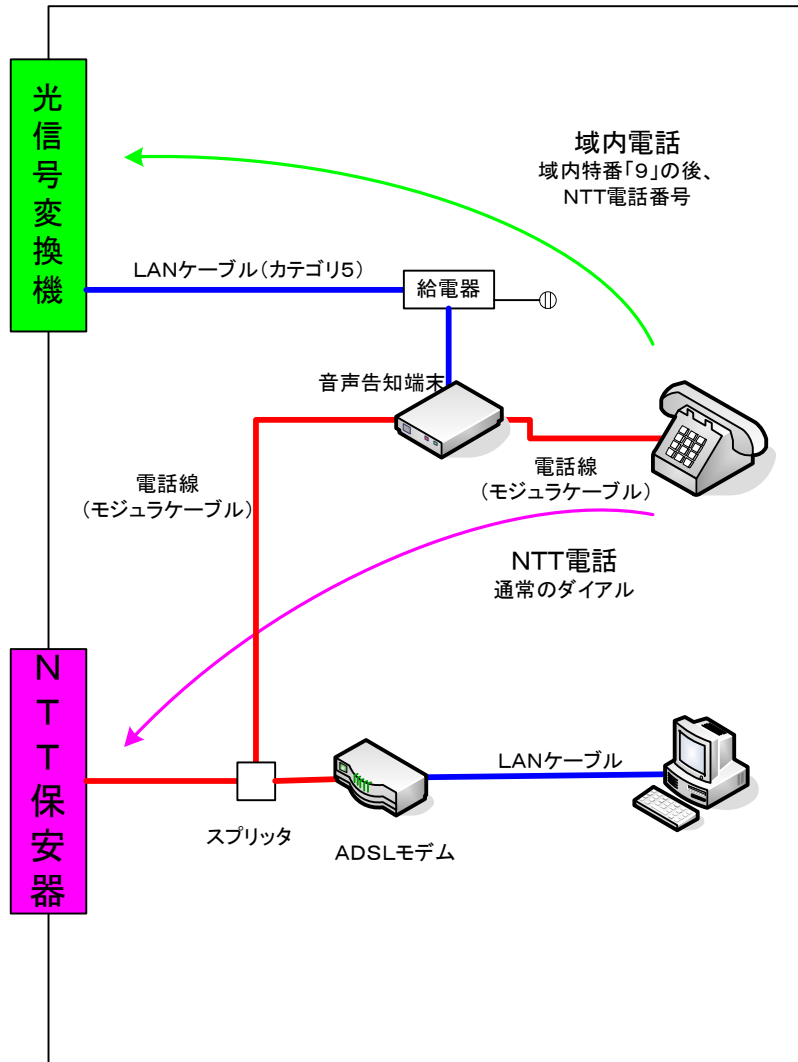
ADSL<インターネットのみ利用> (NTT・域内併用電話の場合)
